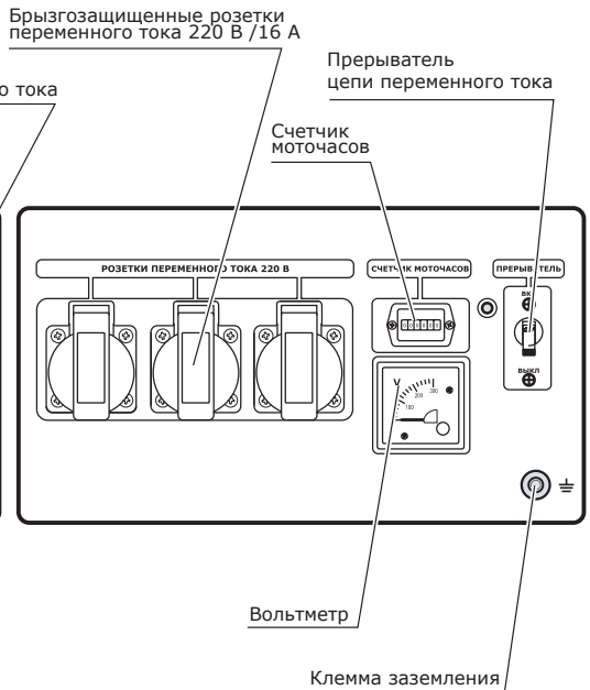
Рис. 10. Схема панели управления генератора УГД-5300 Basic
